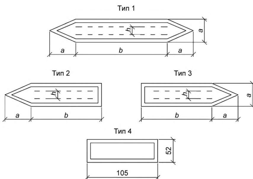
Рисунок 3 — Маркировочные щитки
