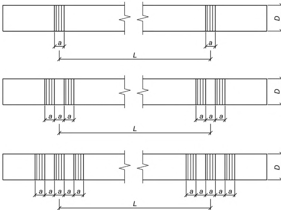
Рисунок 1 — Предупреждающие кольца
